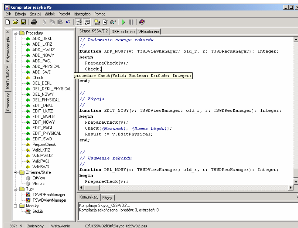
Rys. 3. Środowisko interaktywne kompilatora języka Pascal Script Fig. 3. Integrated Development Environment for Pascal Script
